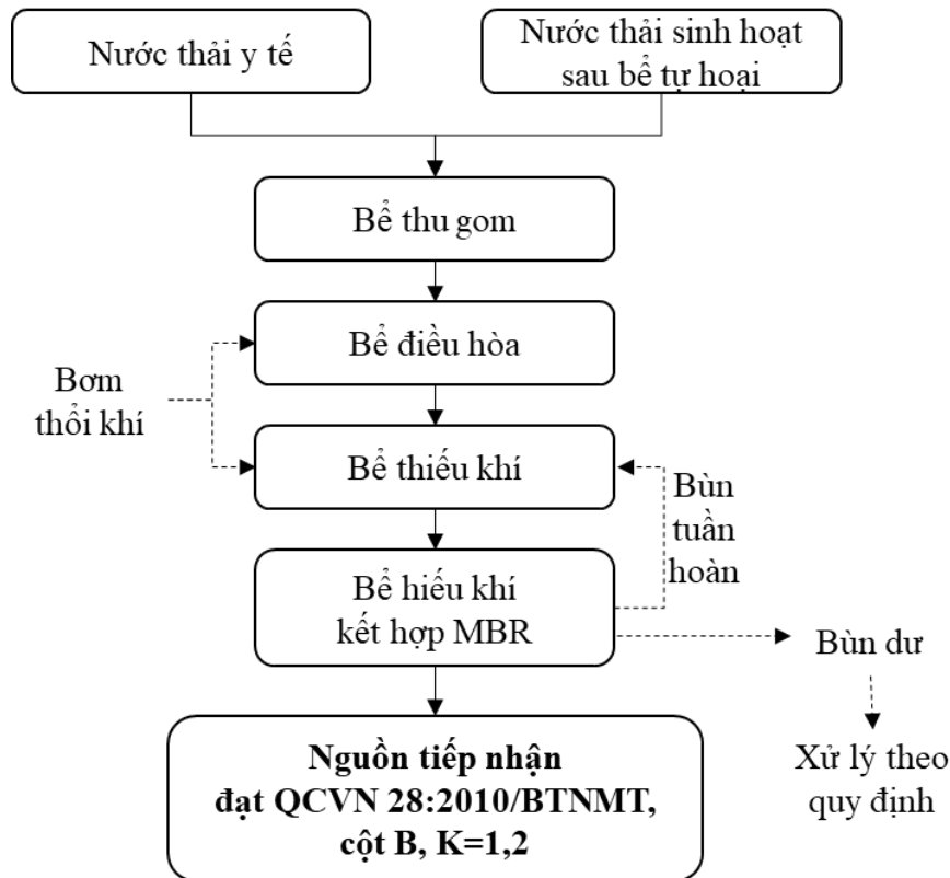
Hình 3.5. Hệ thống xử lý nước thải công suất 10 m 3 /ngày đêm.
