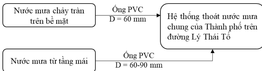
Hình 3.1. Sơ đồ thu gom, thoát nước mưa tại cơ sở.
