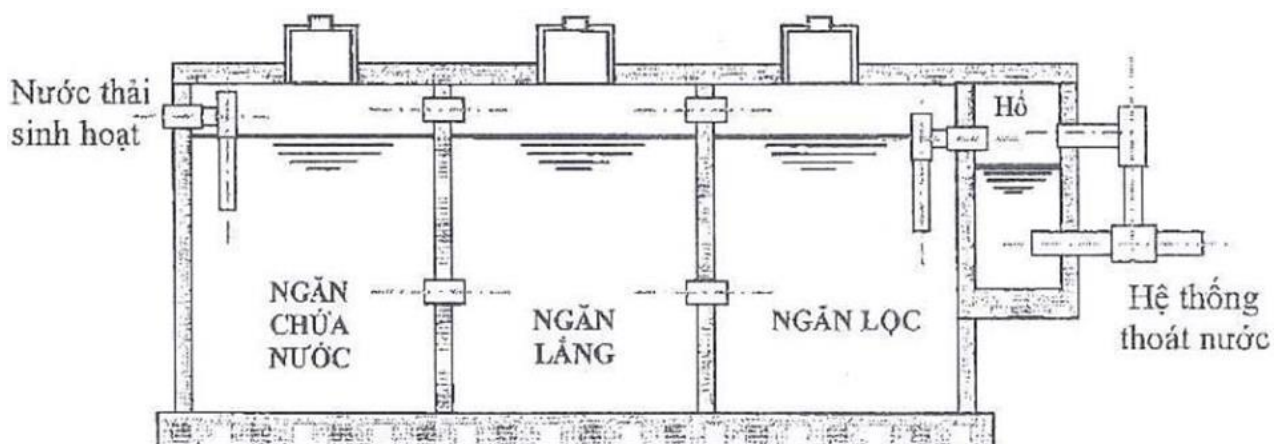
Hình 3.4. Mô hình cấu tạo bể tự hoại 3 ngăn.
