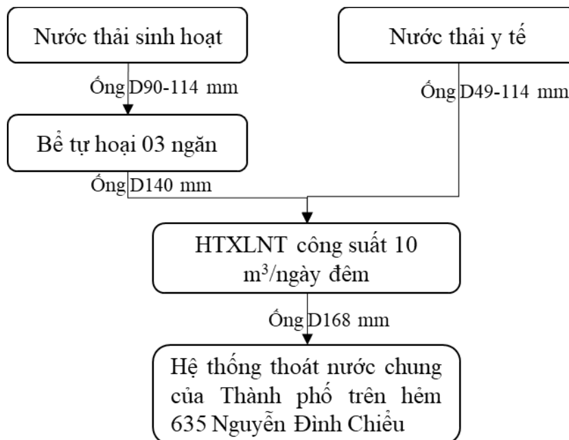
Hình 3.3. Sơ đồ thu gom nước thải tổng quát tại cơ sở.
